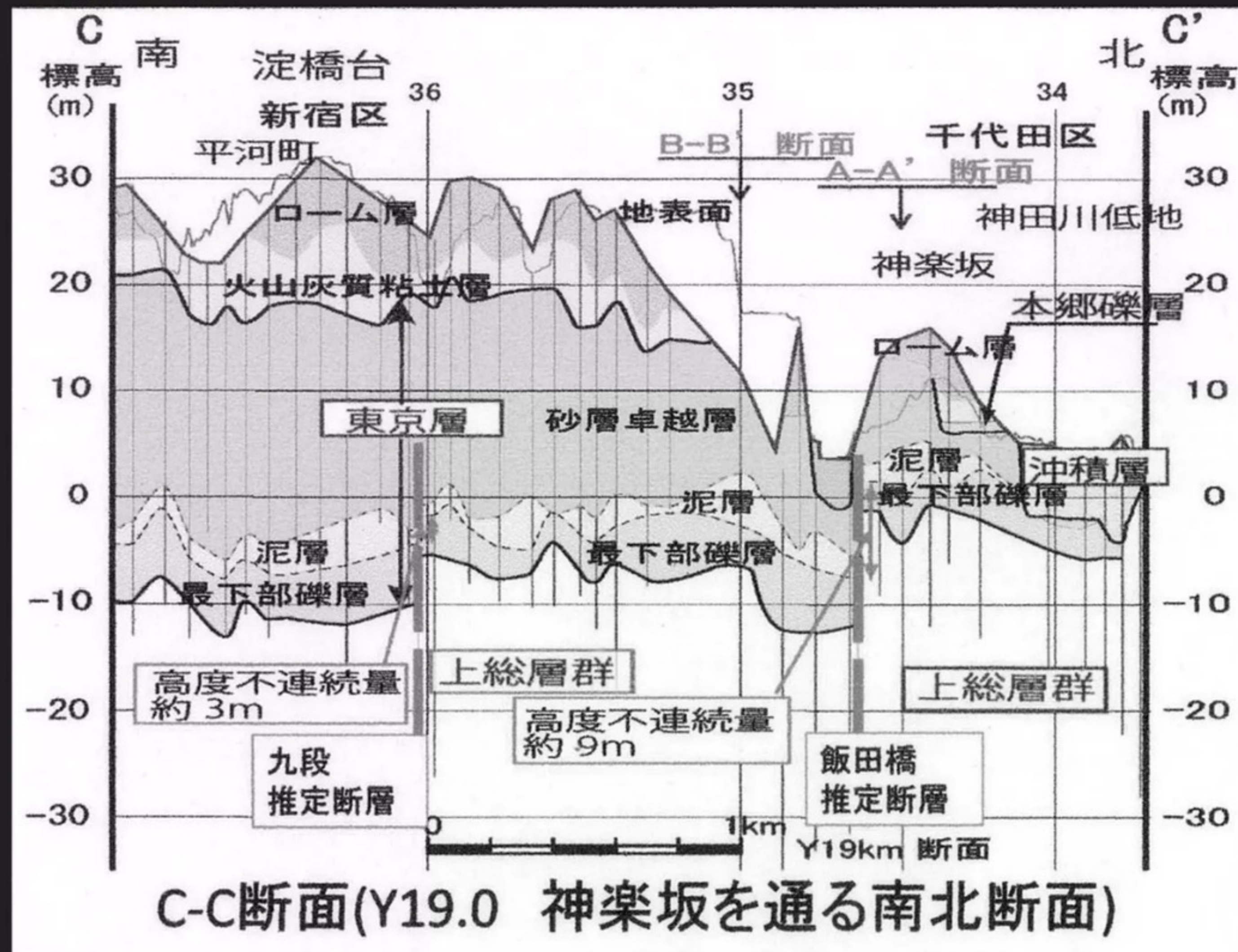
東京都心直下の地層は深部の東京礫層の上に、東京層(20万年程度前)、砂礫層(7~8万年前)、ローム層(7~8万年前から現代)と重なっていて、年代の古い地層ほどずれが大きい(下の図)。この地層断面図では神楽坂を通る飯田橋推定断層と半蔵門駅付近を通る九段断層が過去に地震を繰り返してきたことが推測される(上の図)
